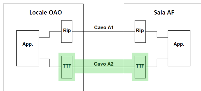
Figura 1: componenti impiantistiche relative al servizio di raccordo passivo in fibra ottica nel tracciato da locale OAO a sala AF
