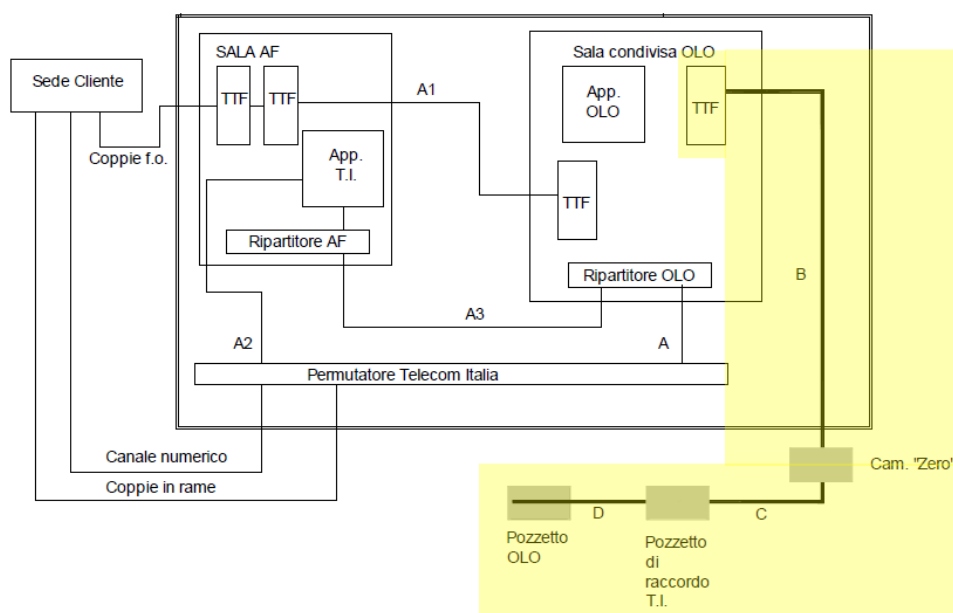
Figura 6: componenti impiantistiche relative al servizio di accesso da cameretta “zero”
