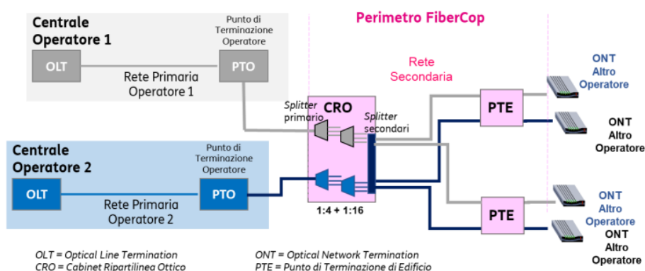
Figura I. 1 - Architettura della rete FTTH di FiberCop
