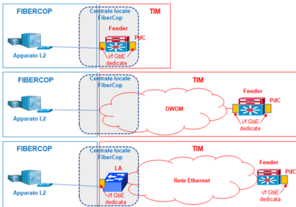
Figura I. 8 - Confini tra perimetro FiberCop e TIM per servizi terminating
