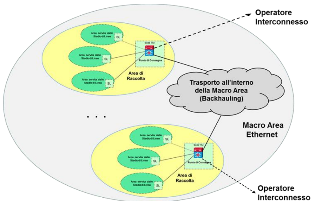
Figura I. 9 – Architettura di raccolta dei circuiti terminating Ethernet su fibra ottica
