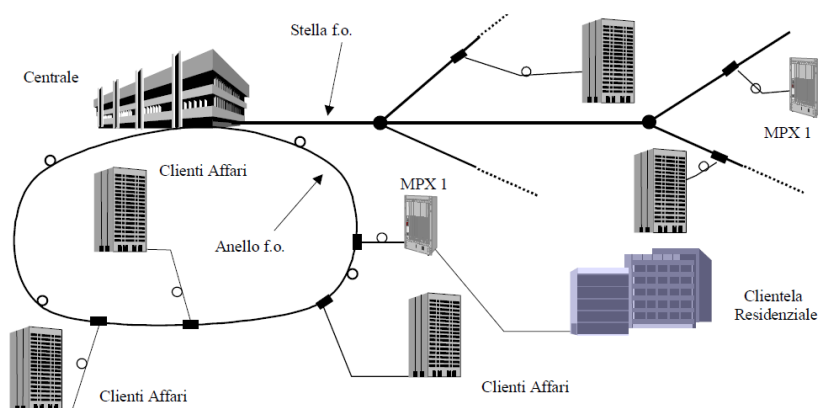
Figura I. 7 – Rete di accesso di FiberCop
