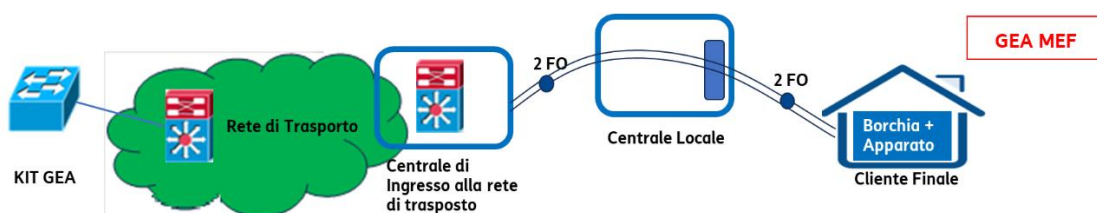
Figura I. 11 - Schema impiantistico del servizio GEA
